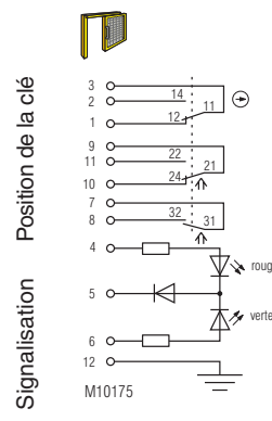
Fig. 2 : Verrouillage à l'état désactivé: 1 re Clé insérée, 2 e Clé à retirer
