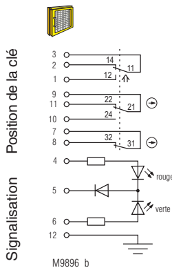
Fig. 1 : Verrouillage à l'état activé: 1 re Clé à retirer 2 e Clé insérée, porte fermée
