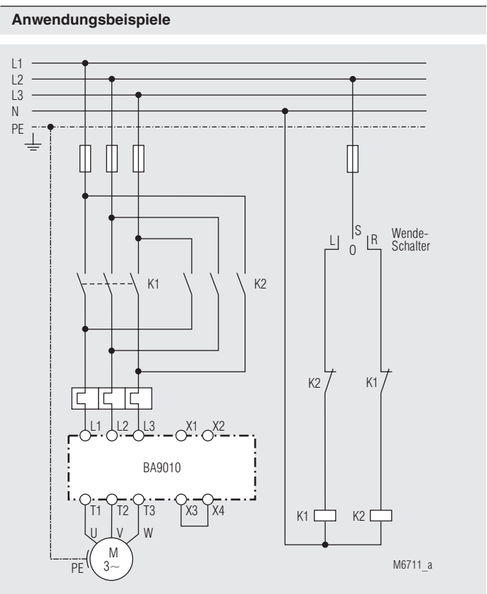
Sanftanlauf mit Reversiermöglichkeit des Motors
