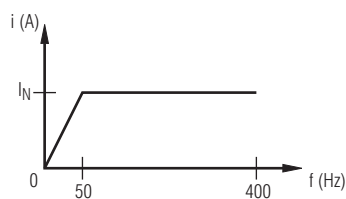
Eingangsstromgrenzkurve in Abhängigkeit von der Frequenz
