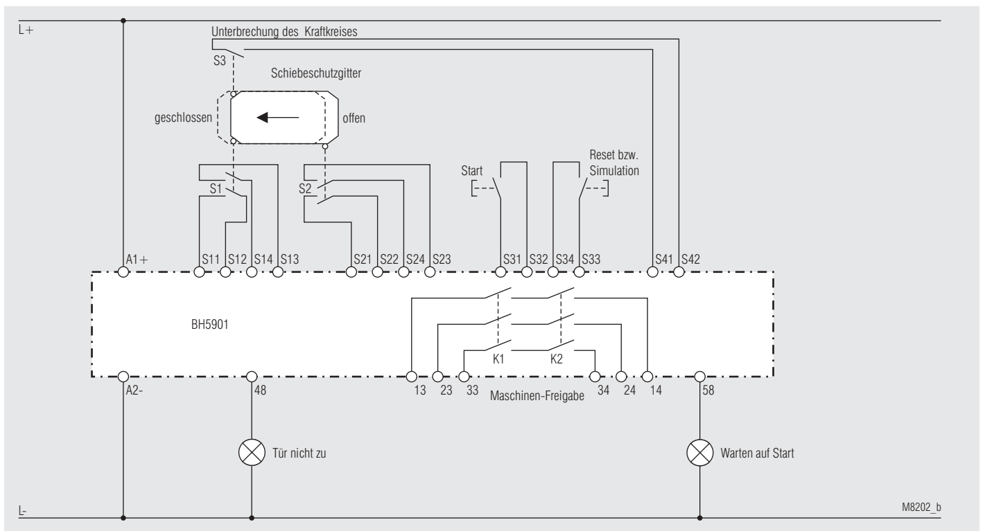
Schutztürüberwachung mit je 2 Schließern als Positionsschalter S1 und S2 für die Türüberwachung und 1 Schließer zur Überwachung des Positionsschalters S3 für die Kraftkreisunterbrechung. (Poti 1: Stellung 2)
