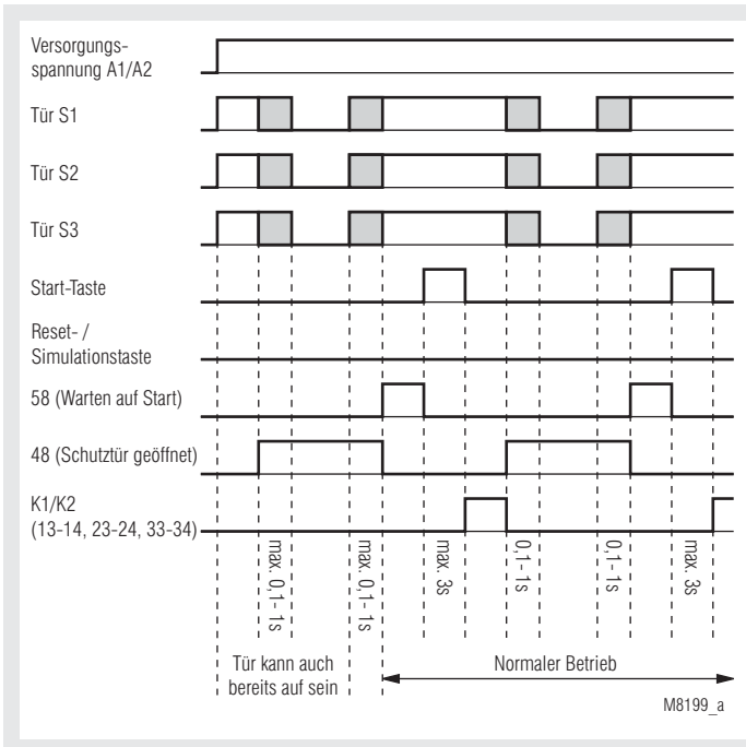
Startsequenz mit Schutztürbewegung
