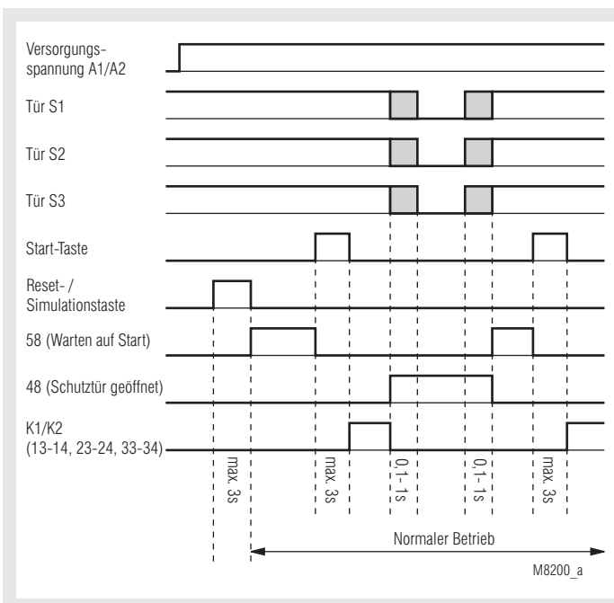
Startsequenz mit Betätigung der Simulationstaste
