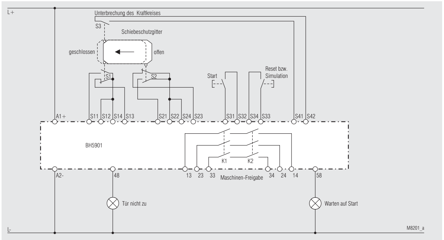
Schutztürüberwachung mit je 1 Wechsler als Positionsschalter S1 und S2 für die Türüberwachung und 1 Schließer zur Überwachung des Positionsschalters S3 für die Kraftkreisunterbrechung. (Poti 1: Stellung 0)
